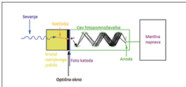
Poenostavljena shema delovanja scintilacijskega detektorja (vir: prirejeno po http://www.physics.isu.edu/radinf/naidetector.htm )
