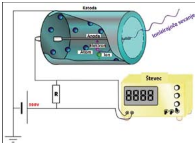
Poenostavljena shema delovanja Geiger-Müller števca (vir: prirejeno po http://www.daviddarling.info/encyclopedia/G/Geiger-Muller_counter.html )
