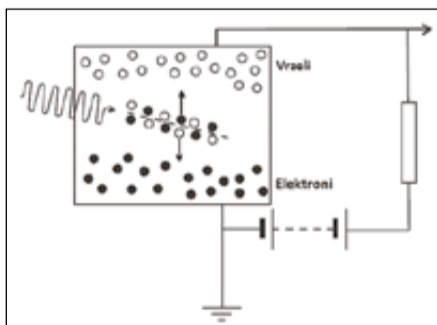
Zelo poenostavljena shema delovanja polprevodniškega detektorja (vir: prirejeno po http://nsspi-apps.ne.tamu.edu/NSEP/basic_rad_detection/index.php?course=0600 )
