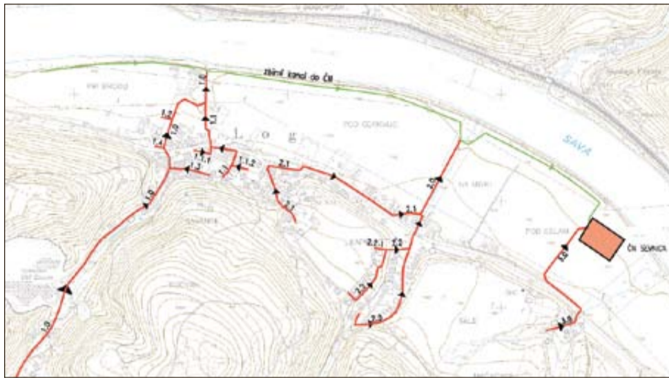
Situacija vodov kanalizacije na Logu (Vir: foto arhiv Občine)
